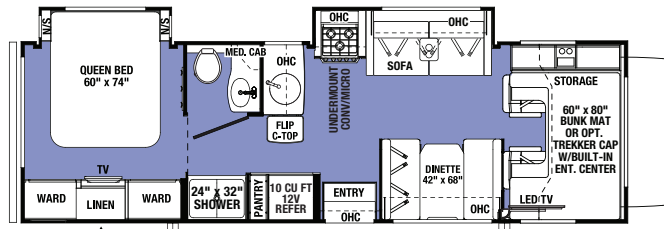
16' AWNING 2860DS (Available on Ford E450/Chevy 4500)
